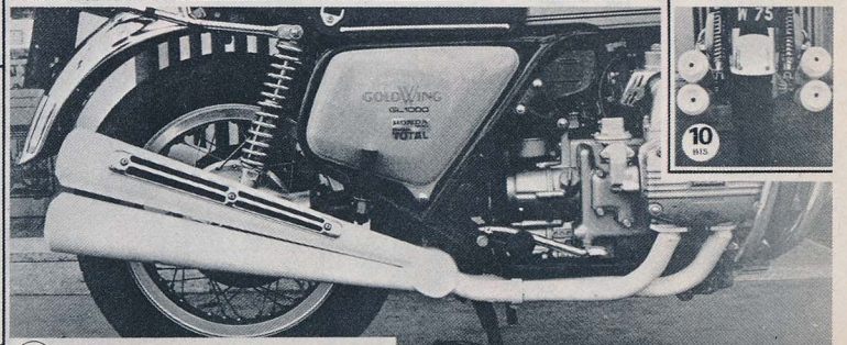
10 Echappement noir mat "1004 PRESTIGE" pour GL 1000
