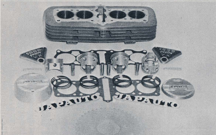
5 Kit moteur 1000 VX pour CB 750
