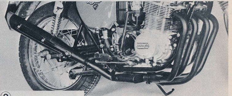
9 Echappement 4 dans 1 pour CB 500 et 750
