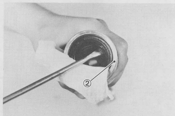
—72— 2. Oil seal 2. Bague d'étanchéité
